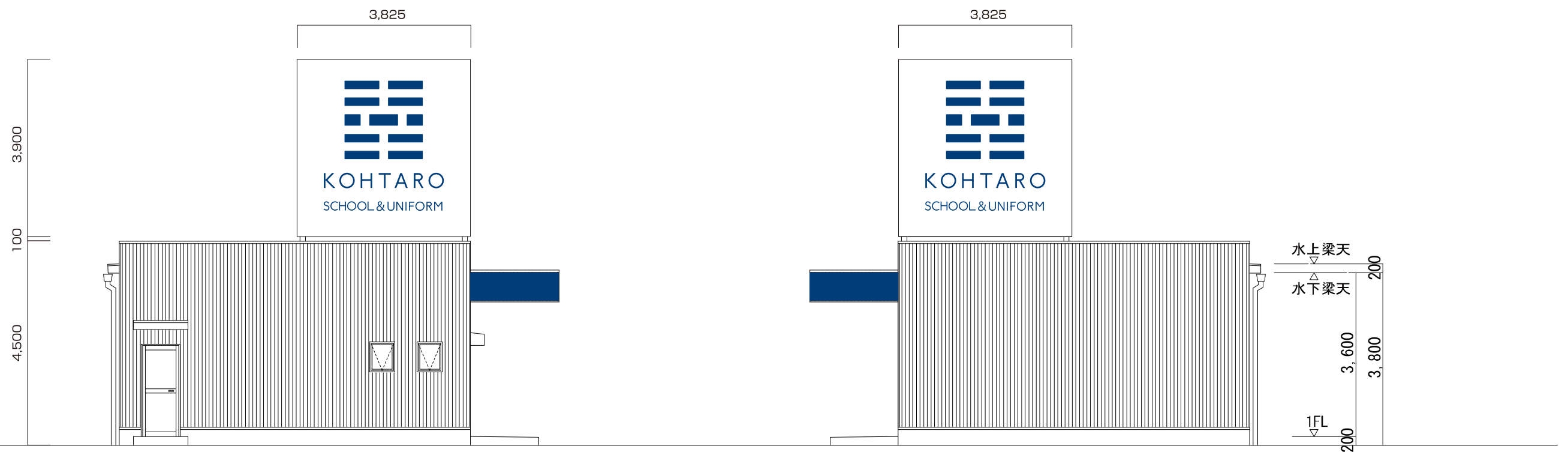
東面 立面図 S=1/100
